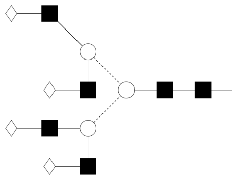
Oxford Notation
