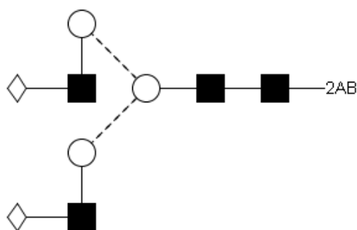
Oxford Notation
